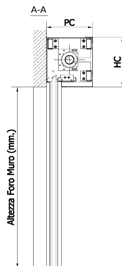
Schema di installazione Tipo 1
