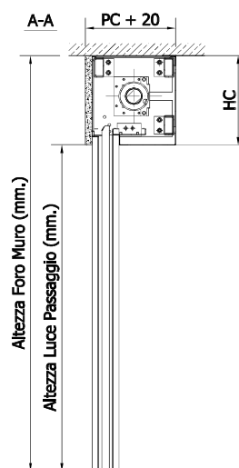
Schema di installazione Tipo 2
